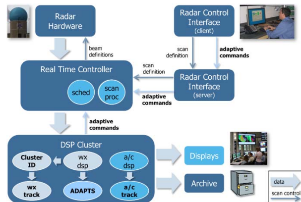
Fig. 1. NWRT PAR functional diagram.
